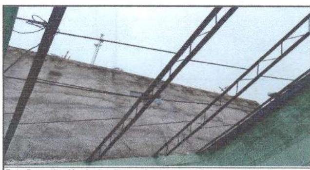
Foto 5: sustitución de duralita por lamina troquelada calibre 26 y mantenimiento de soporte de metal
